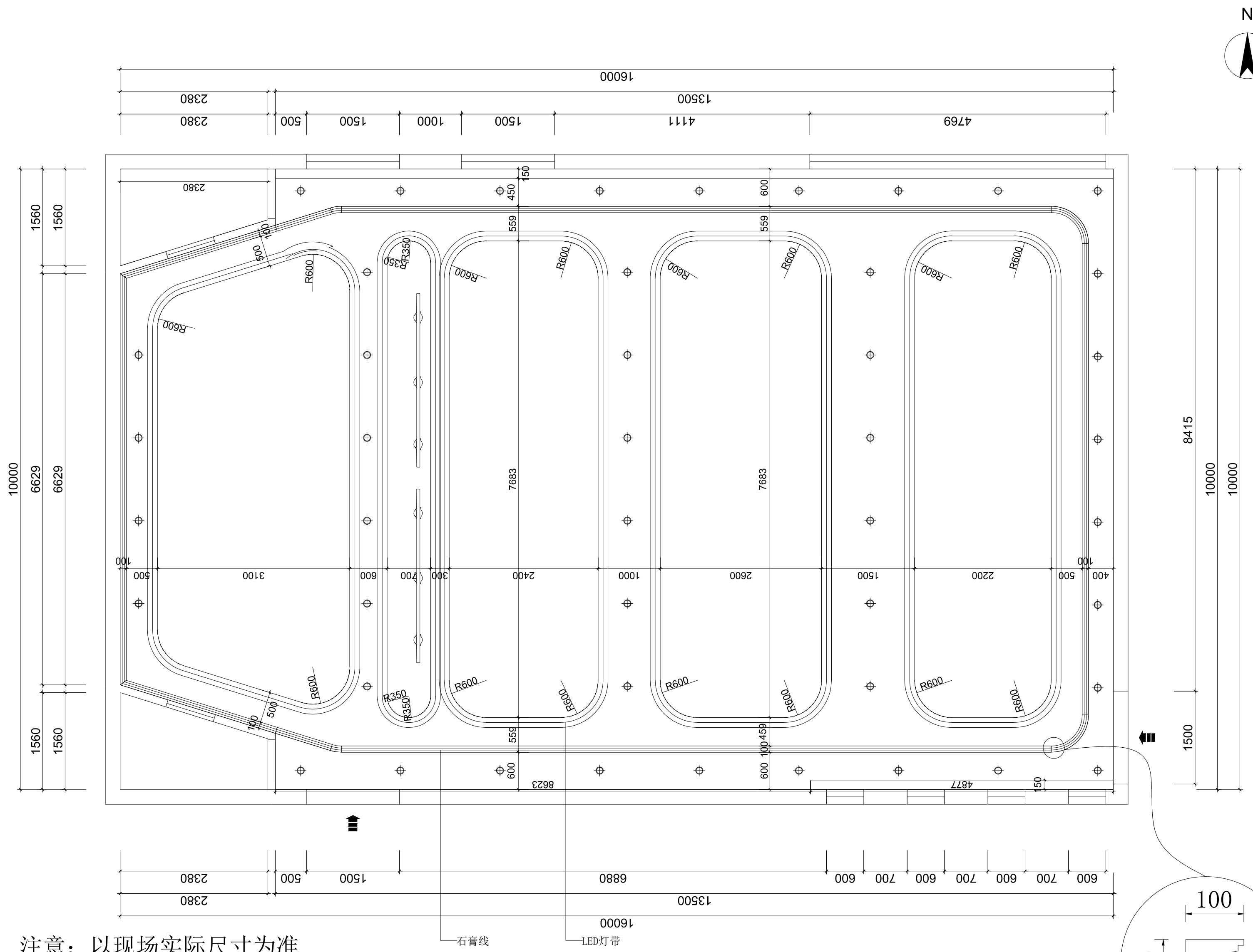
天花尺寸(1:100)
